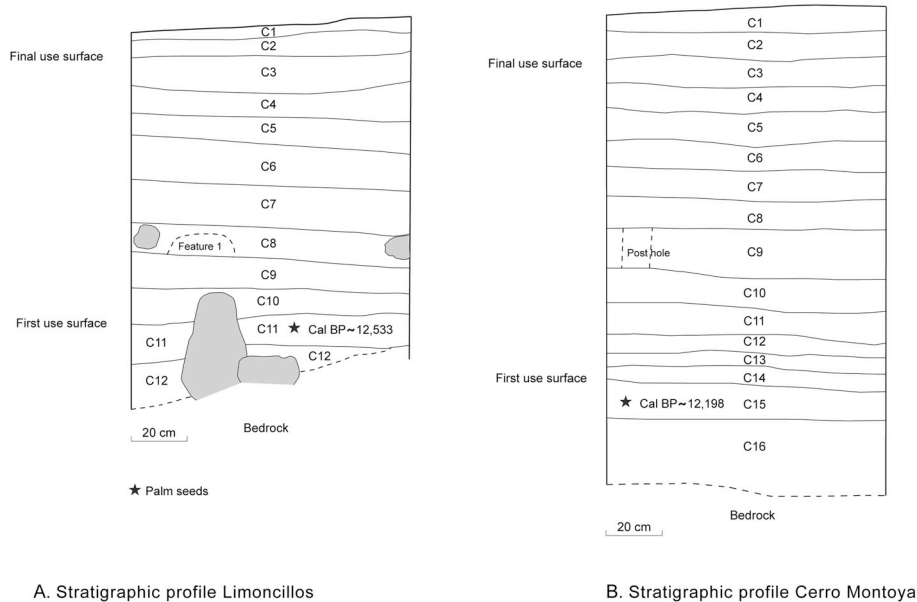
Fig. 5. Stratigraphic profiles. A. Limoncillos; B. Cerro Montoya.
